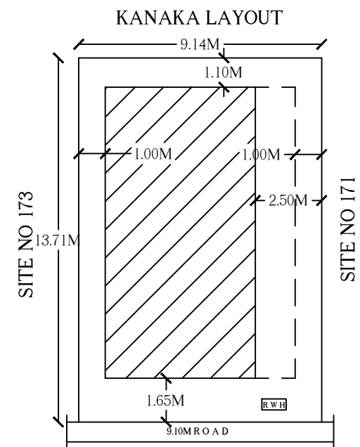
SITE PLAN 1:200
